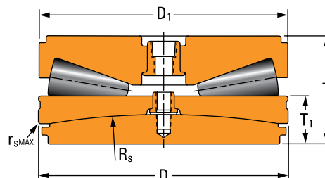
Fig. 96. Type TTHDFLSV-2.
