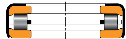
Fig. 14. Type TTSP.
