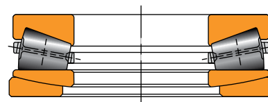
Fig. 11. Type TTHDFLSA.
