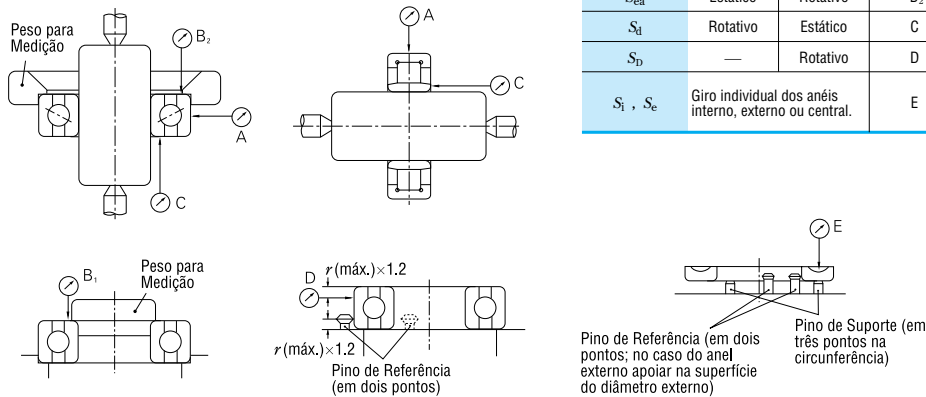
Fig. 8.1 Métodos de Medição da Precisão de Giro (simplificado)
