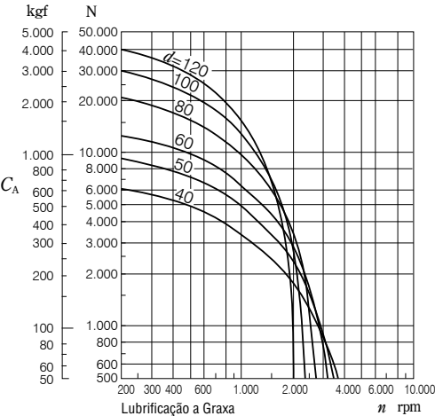
Fig. 5.13 Carga Axial Permissível nos Rolamentos de Rolos Cilíndricos Para rolamentos da série de diâmetro 3 ( k=1,0 ) em carregamento contínuo e lubrificadas com graxa ou óleo.
