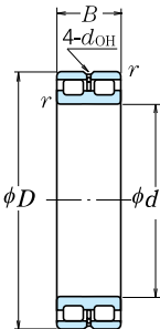
Rolamento Lado Livre Tipo RSF
