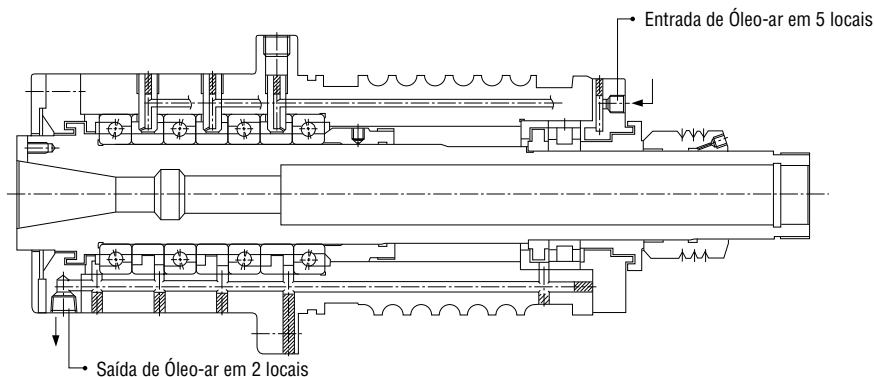
Fig. 12.10 Lubrificação Óleo-ar
