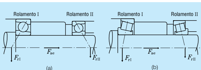
Fig. 5.12 Cargas Atuantes nos Rolamentos Contrapostos
