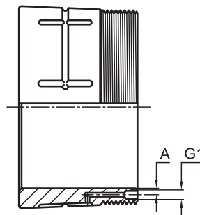
BUCHA DE FIXAÇÃO HE, HA, HS COM MS REPRESENTAÇÃO DA CANALETA DE ÓLEO PARA BUCHAS HIDRÁULICAS OHE ....H, OHA ....H, OHS ....H
