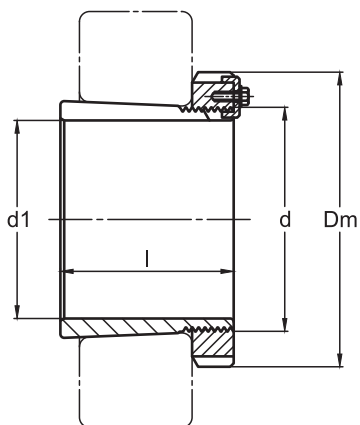
REPRESENTAÇÃO DA CANALETA DE ÓLEO PARA BUCHAS HIDRÁULICAS OHE ....H, OHA ....H, OHS ....H
